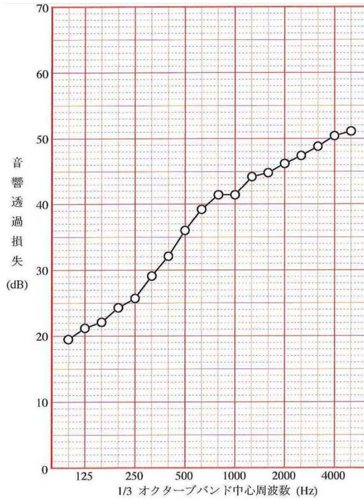
音響透過損率
