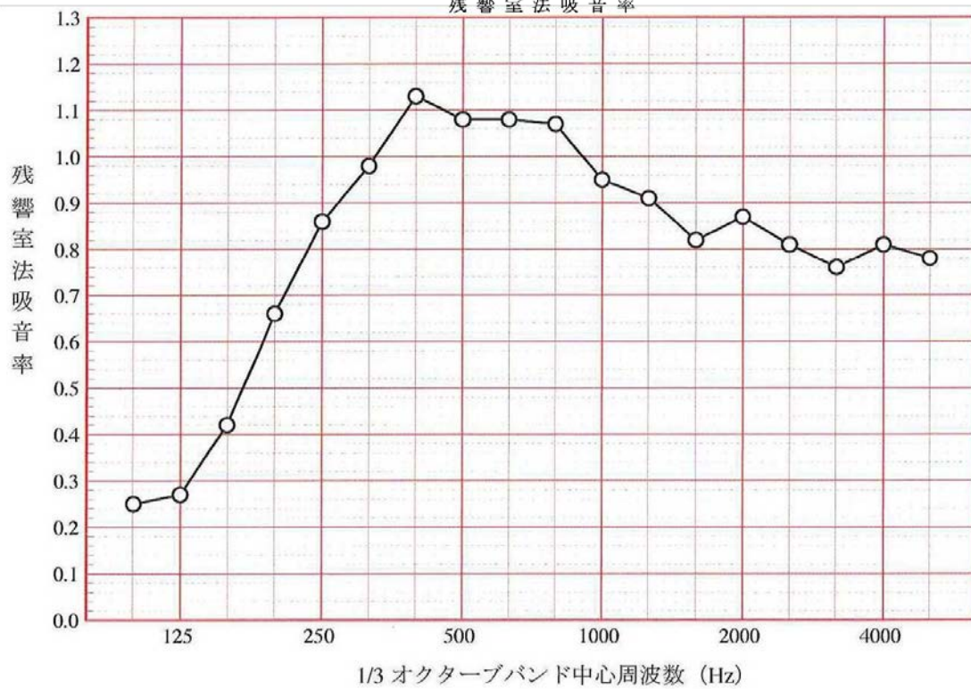
残響室法吸音率
