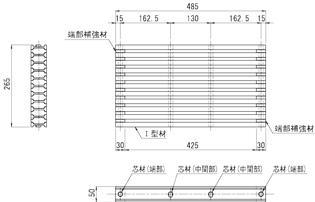
FRP製トンネル用マス蓋 詳細図 S=1:5
