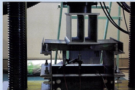
・設計荷重100kNによる載荷重試験
