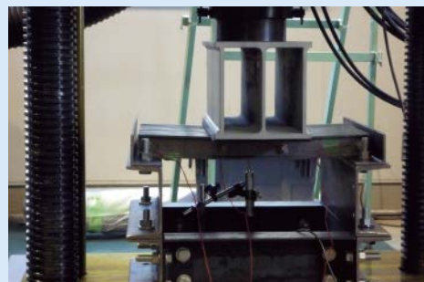
・設計荷重53kNによる載荷重試験
